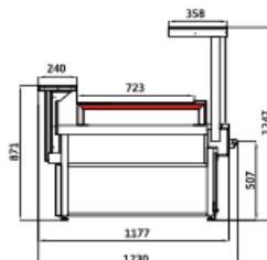
VOGTLAND HP mit heißer Platte
