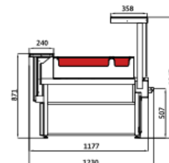
VOGTLAND HW mit Wasserbad
