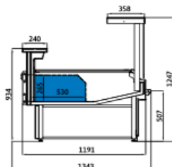
VOGTLAND FG mit Unterbaukühlung
